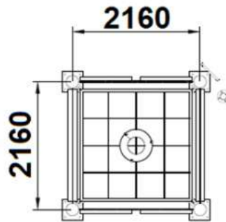
A-A SECTION
