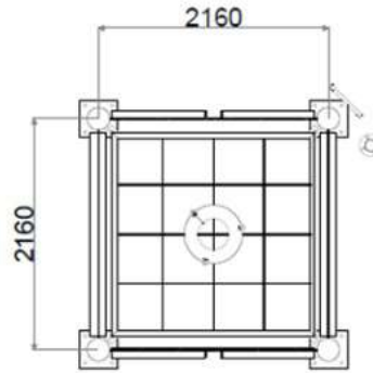
A-A SECTION
